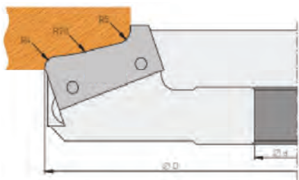
Profil: 47000310 40 x 20 x 2mm
