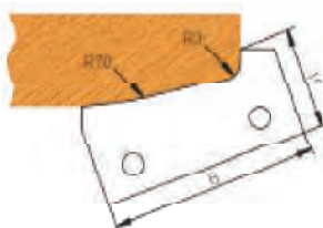
Profil: 47000312 40 x 20 x 2mm
