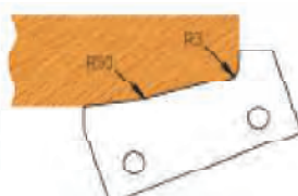
Profil: 47000313 40 x 20 x 2mm
